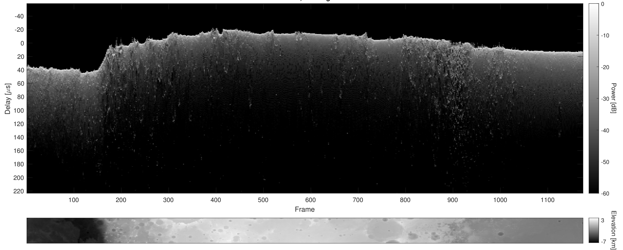
Orbit 8176, Cluttergram
